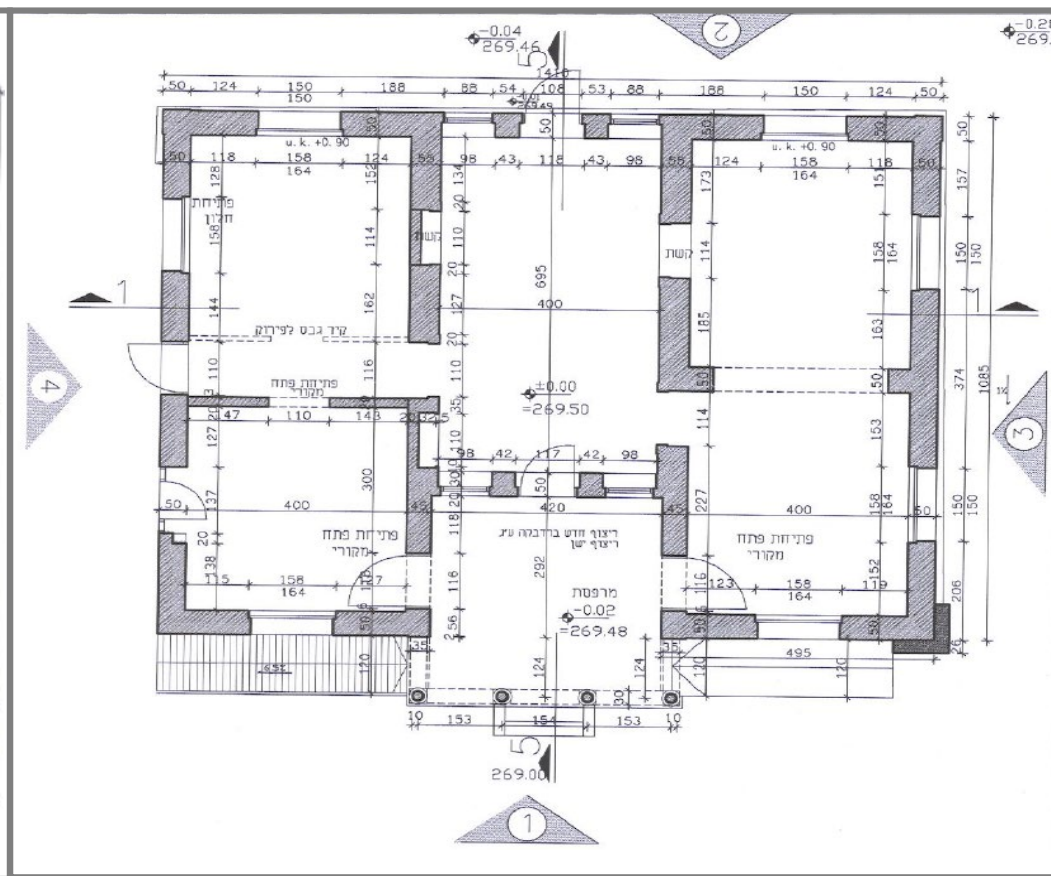
תוכנית קרקע - מצב מקורי
