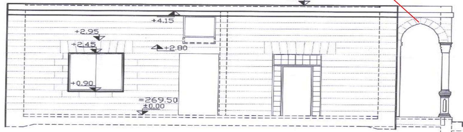
4 חזית דרום מערב
