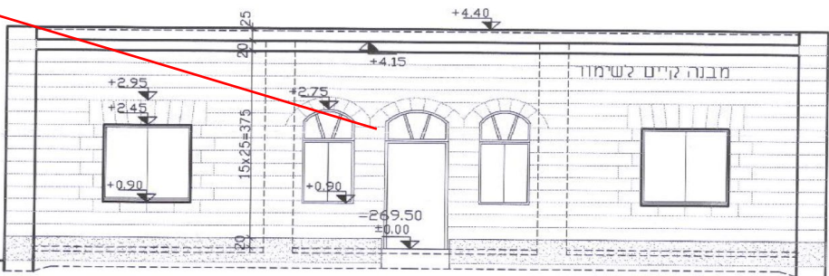
חזית צפון מערב 2
