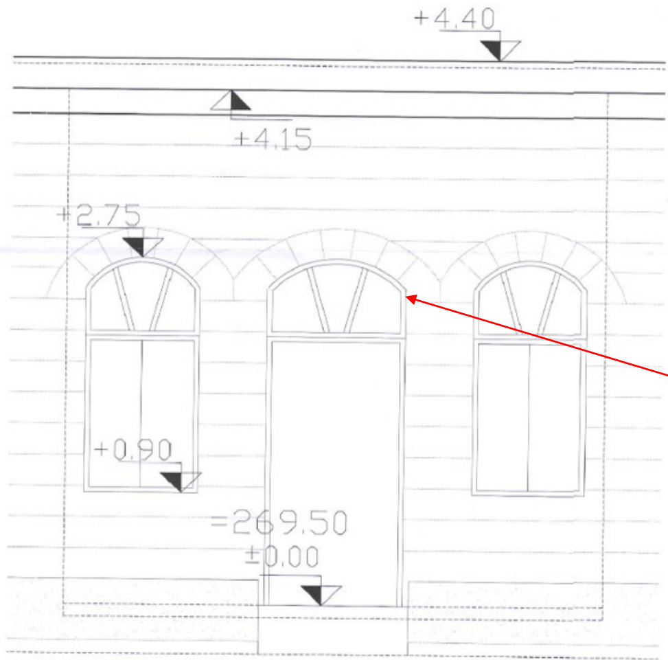
קטע חזית אחורית 1:25
