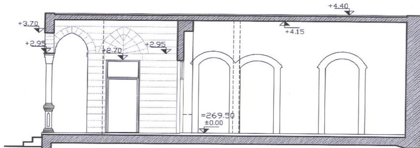
חתך 5 - 5
