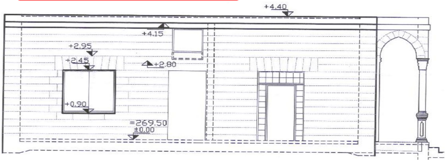
חזית דרום מערב ④
