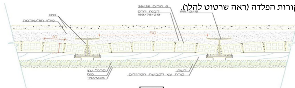
כנים חתך טיפוסי של תקרה
