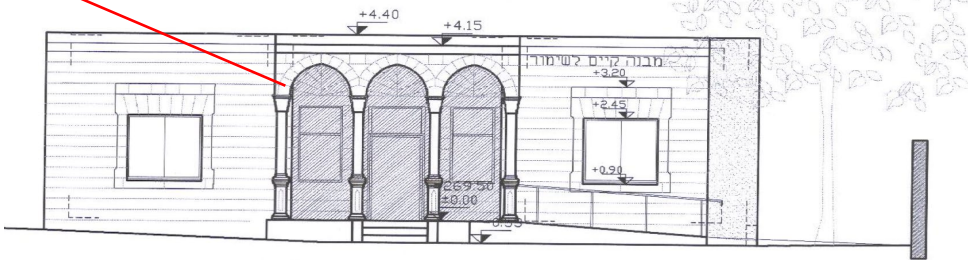
חזית דרום מזרח 1
