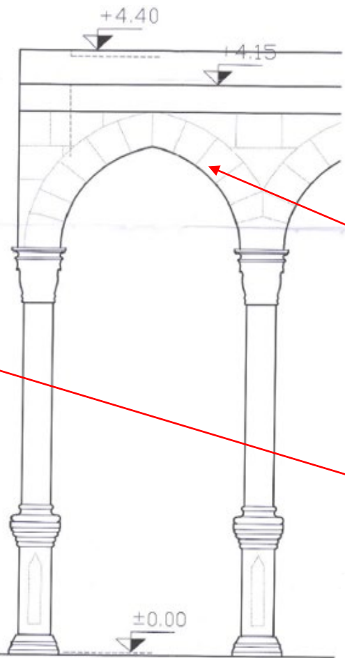
קשתות בכניסה 1:25
