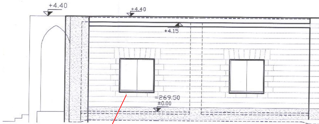
3 חזית צפון מזרח
