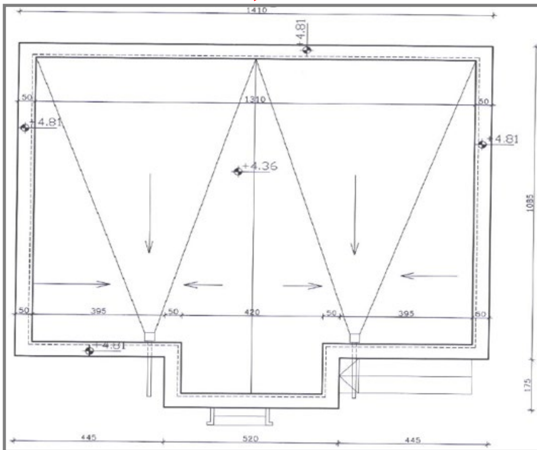
תוכנית גג - מצב מקורי
